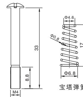
安装螺丝
